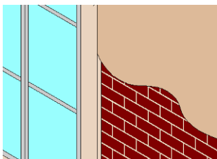
La surface de l'enduit et les éléments apparents (ici encadrement de baie) sont sur un même plan. Les maçonneries sont en retrait pour tenir compte de l'épaisseur de l'enduit.
